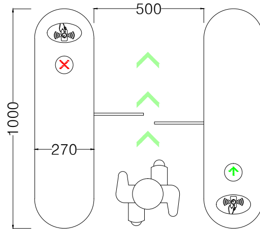
HCT 270-S TEKNİK ŞEMA
